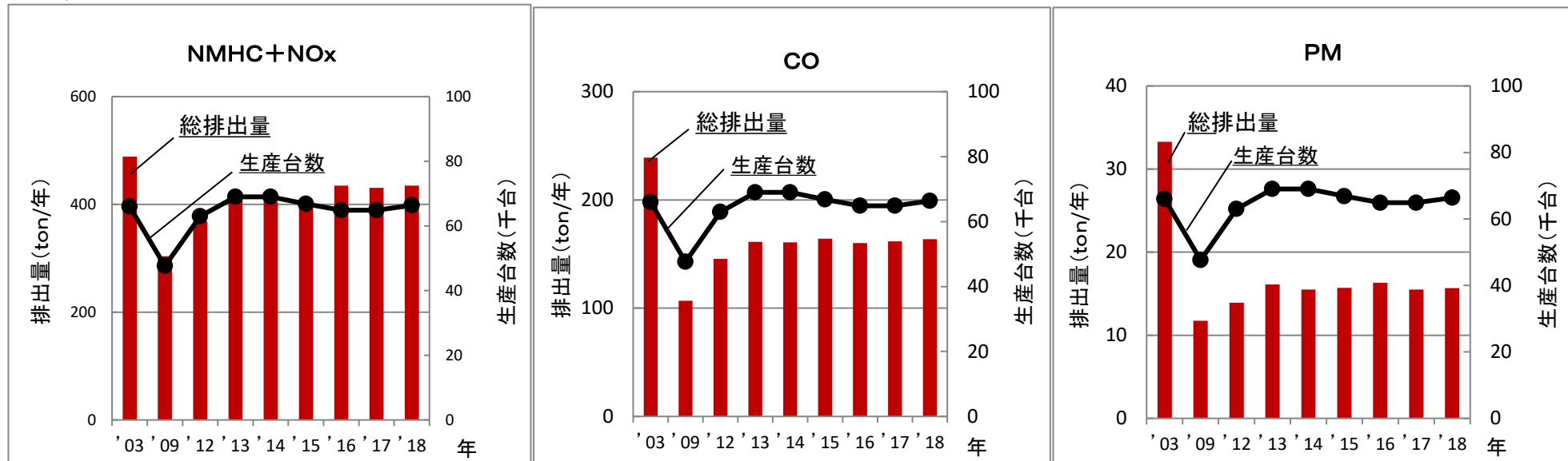
図1. ディーゼルエンジン排出ガス量（2018年）
